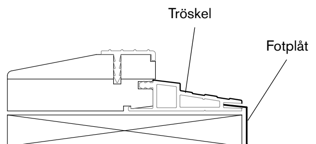
Montering med karmskruv
