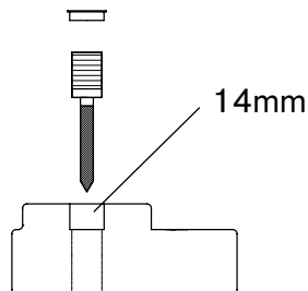
Montering med karmskruv
