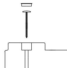
Montering med skruv
