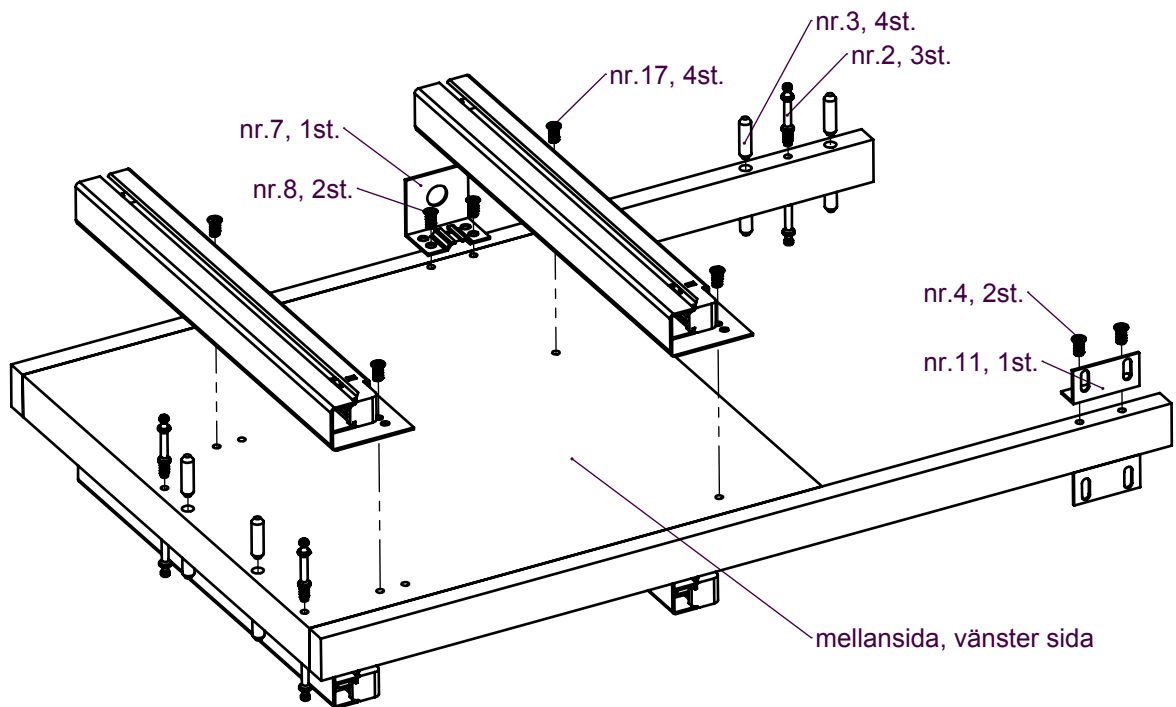
Monterad mellansida Vy vänster sida
