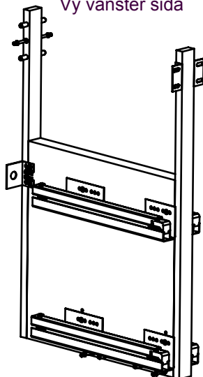
Monterad mellansida Vy vänster sida
