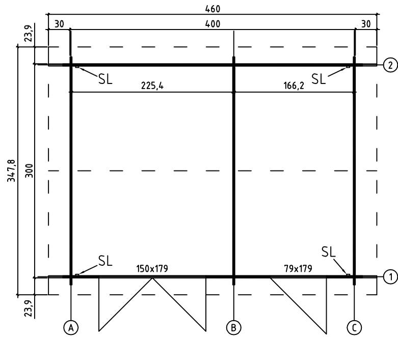
GROUNDPLAN - GRUNDPLAN - PLAN DE MASSE
