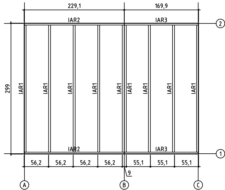
FOUNDATION - FUNDAMENT - FONDATION
