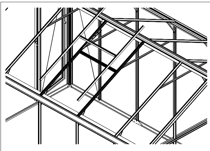
SE - Montera gummilister NO - Montere gummilister FI - Asenna kumitiivisteet DK - Monter gummilister UK - Install rubber seals
