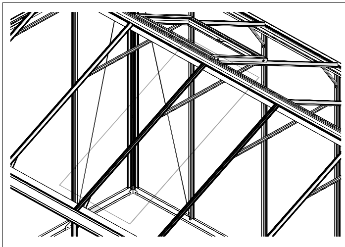
SE - Demontera glas (spara/återvinne) NO - Demontere glass (spare/gjenvinne) FI - Irrota lasi (sästä/kierrätä) DK - Afmontere glas (gem/genanvend) UK - Remove glass (save/recycle)
