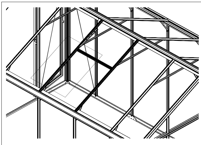
SE - Montera glas (604) NO - Montere glass (604) FI - Asenna lasi (604) DK - Monter glas (604) UK - Install glass (604)
