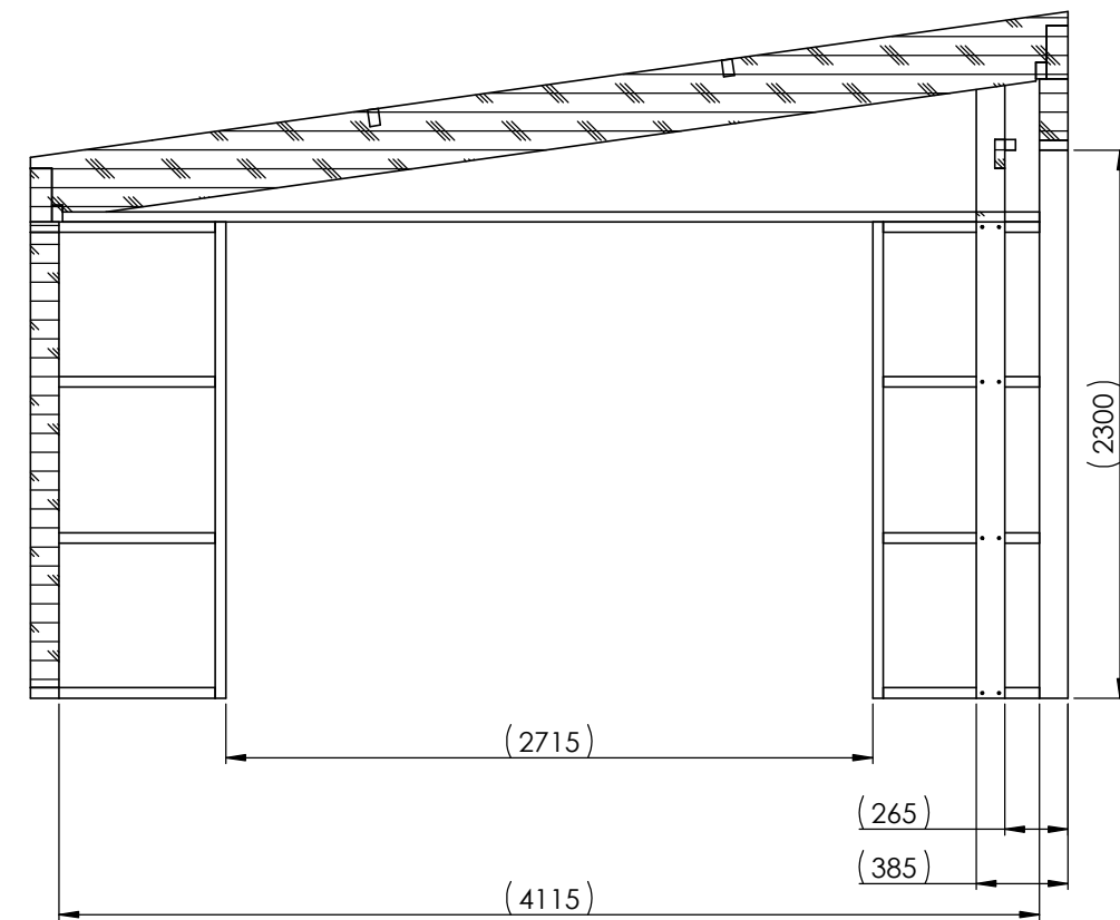
SECTION A-A
