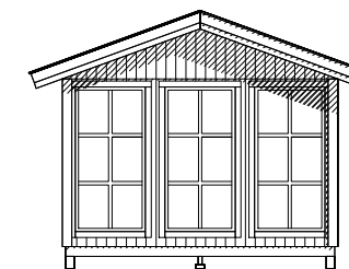
FASAD MOT
