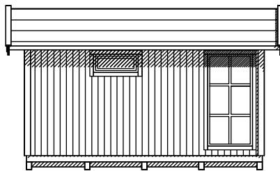
Långsida
