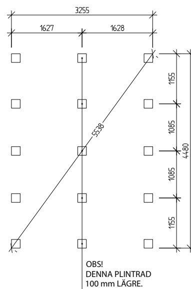
Plintritning
