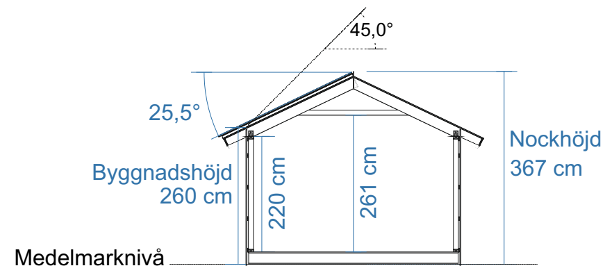
SEKTION
